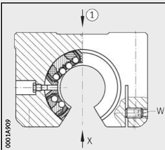
KTSOS...-PP-AS
