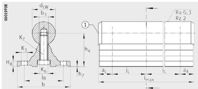
TSNW..-G4, TSNW..-G5
