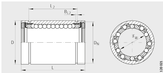
KB
