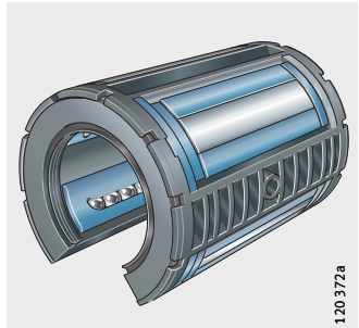
KTSG...-PP-AS, KTSS...-PP-AS
