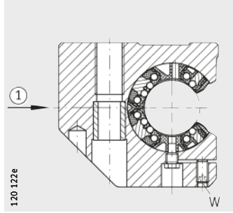
KGSCS...-PP-AS ① 8)
