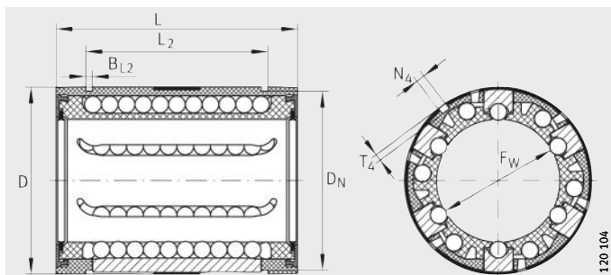
KN..-B-PP, KN..-B
