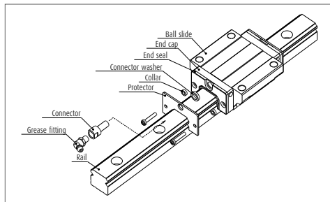
Fig. 13 Protector
